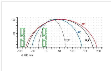
Tafelzaag TS 161/21
