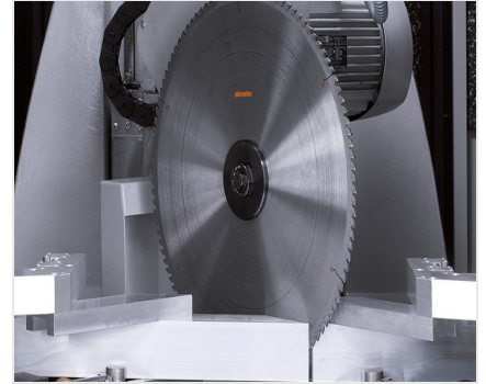
Profielbewerkingscentrum SBZ 631
