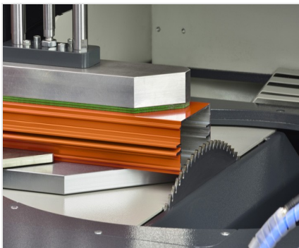
Zaagcentrum SBZ 616/02
