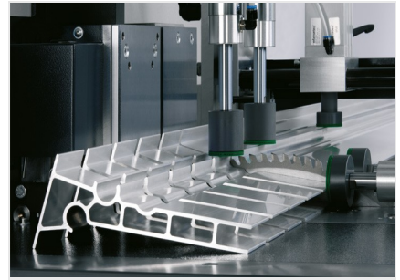
Zaagautomaat SAS 142/44
