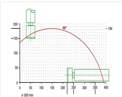
Zaagautomaat SAS 142/43
