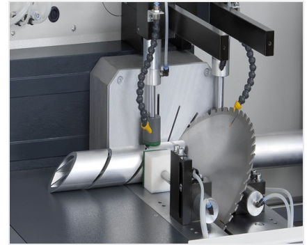
Zaagautomaat SAS 142/43
