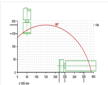
Zaagautomaat SAS 142/43
