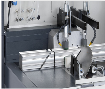
Zaagautomaat SAS 142/43
