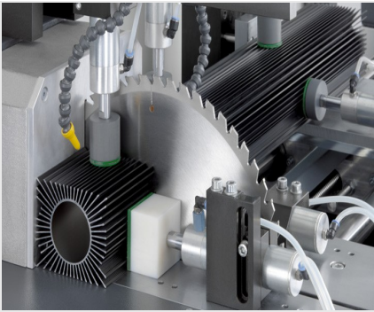
Zaagautomaat SAS 142/43
