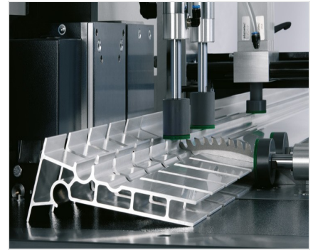
Zaagautomaat SA 142/38
