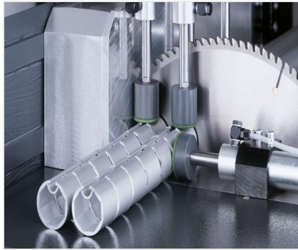
Zaagautomaat SA 142/37
