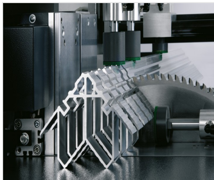
Zaagautomaat SA 142/38
