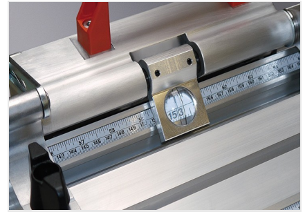
Aanslag- en meetsysteem MMS 200
