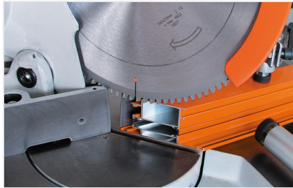
Verstekzaagmachine MGS 73/33
