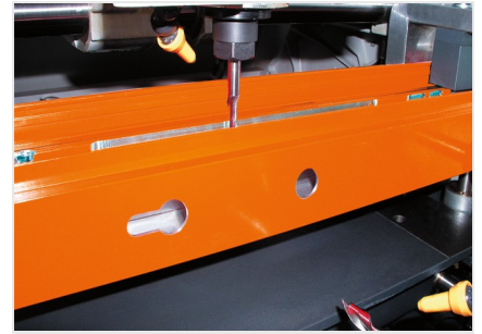
Tweespindel- kopieerfreesmachine KF 78/23
