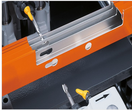
Tweespindel- kopieerfreesmachine KF 78/23
