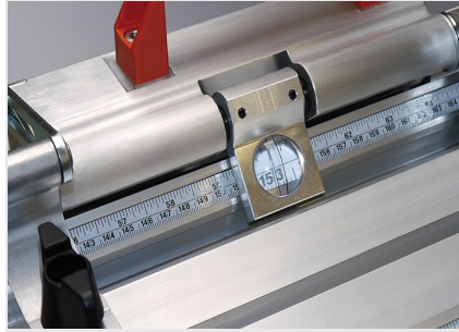
Aanslag- en meetsysteem AMS 200
