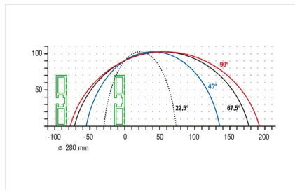
Sega a tavolo TS 161/21
