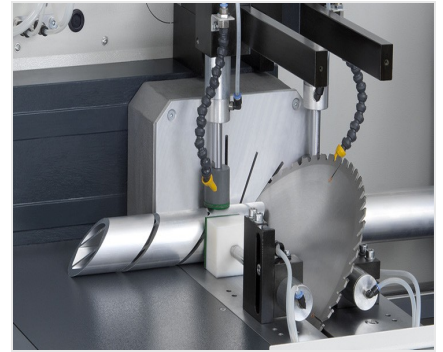
Troncatrice automatica SAS 142/43
