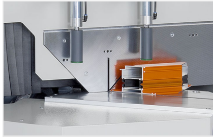
Troncatrice per tagli obliqui MGS 105
