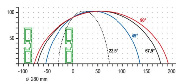
Scie à table TS 161
