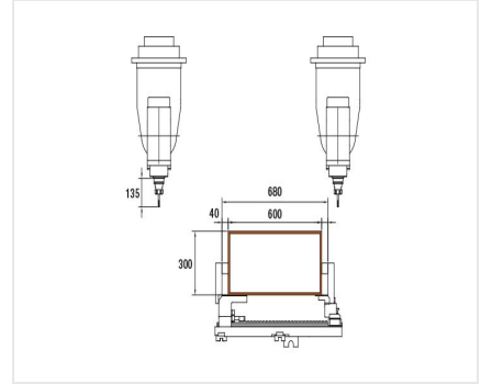
Centre d'usinage de barres SBZ 151 Edition 90
