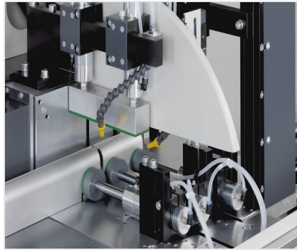
Scie automatique SAS 142/44
