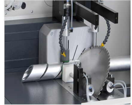
Scie automatique SAS 142/43
