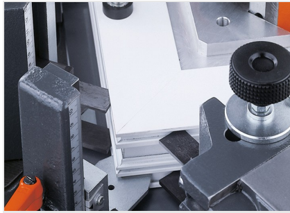
EP 124 Sertisseuse d'angle
