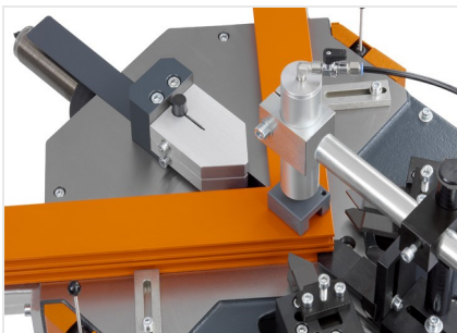
EP 120 Sertisseuse d'angle
