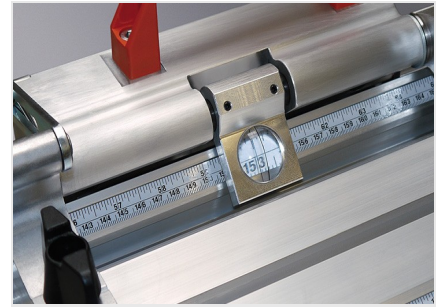
Système de butée et de mesure AMS 200
