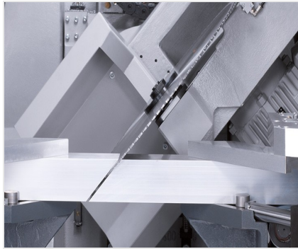
Centro de mecanizado de barras SBZ 631
