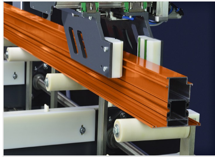
Banco de corte a medida SBZ 616/02
