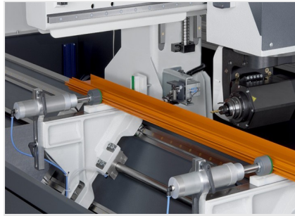
Centro de mecanizado de perfiles SBZ 122/74
