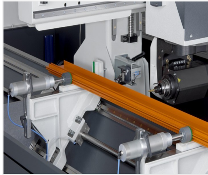
Centro de mecanizado de perfiles SBZ 122/74
