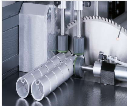
Tronzadora automática SA 142/37
