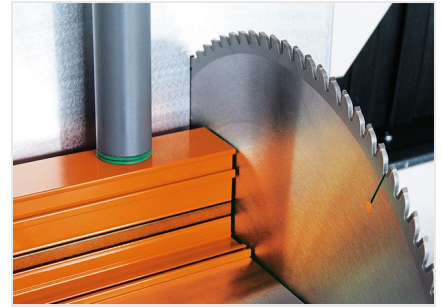
Tronzadora doble DG 104
