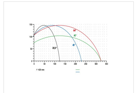
Tronzadora doble DG 104 Diagrama de corte DG 104
