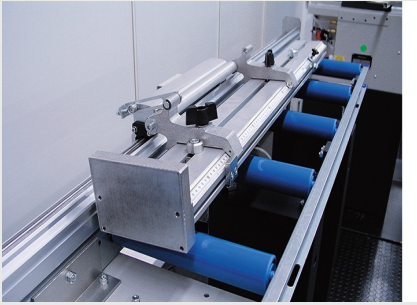
Sistema de tope y medición AMS 200
