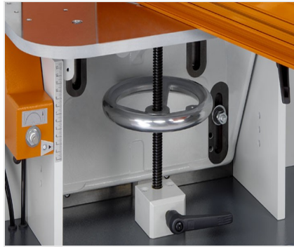
Fresadora retestadora AF 223/01
