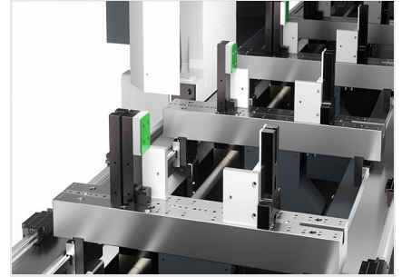
Stabbearbeitungszentrum SBZ 141
