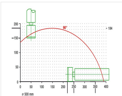
Sägeautomat SAS 142/44
