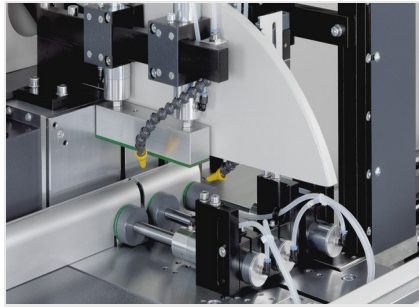
Sägearbeitzeug SAS 142/44
