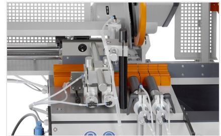
Sägeautomat SA 73/36
