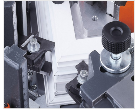
Eckverbindungspresser EP 124
