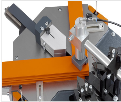
Eckverbindungspresse EP 120
