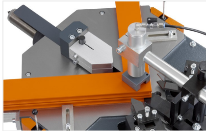
Eckverbindungspressen EP 120
