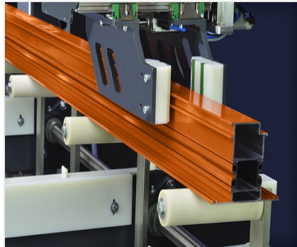
Nářezové centrum SBZ 616/02
