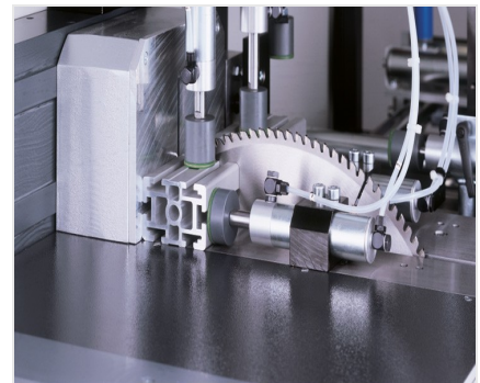
Pilový automat SA 142/37
