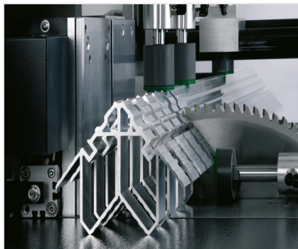
Pilový automat SA 142/38
