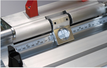
Système de butée et de mesure MMS 100
