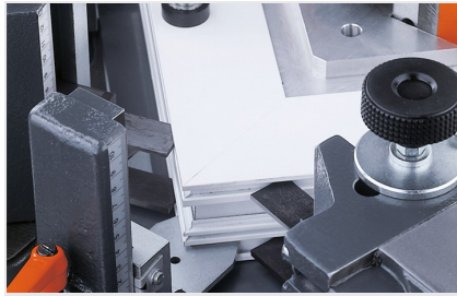
EP 124 Sertisseuse d'angle
