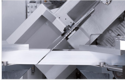
Centro de mecanizado de barras SBZ 631
