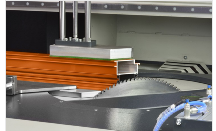
Banco de corte a medida SBZ 616/02
