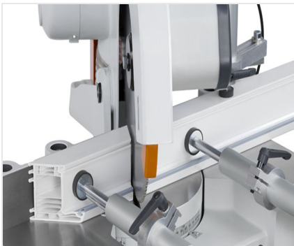
Tronzadora MGS 73/33
