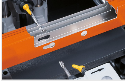
Copiadora fresadora triple KF 178/10
