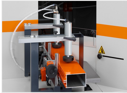
Tronzadora retestadora AKS V-550
