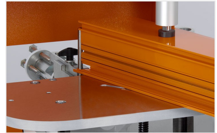
End milling machine AF 223/01
