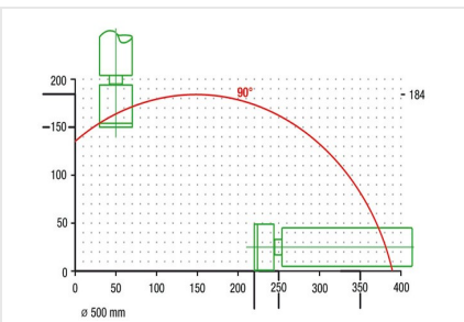
Säageautomat SAS 142/43
