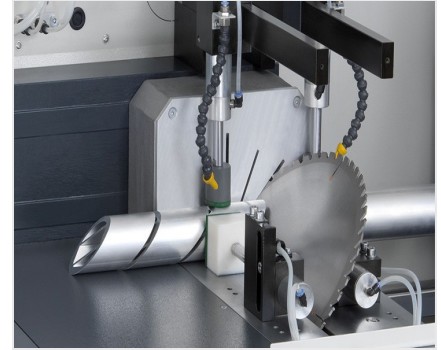
Sägearbeitzeug SAS 142/43
