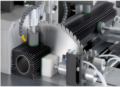
Säageautomat SAS 142/43
