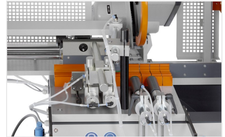
Sägeautomat SA 73/36
