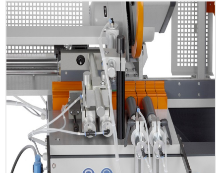
Sägeautomat SA 73/36
