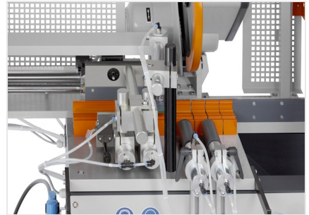
Sägeautomat SA 73/36
