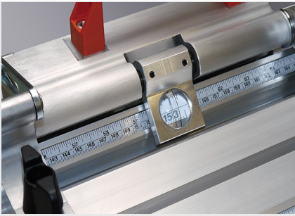
Anschlag- und Mess- System MMS 100
