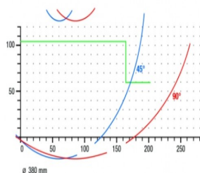
Gehrungssäge MGS 73/33
