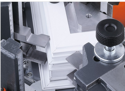
Eckverbindungspresse EP 124
