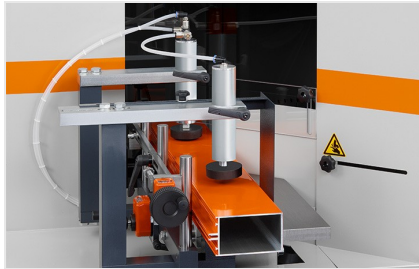
Ausklinksäge AKS V-550
