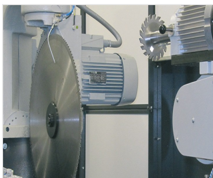
Centrum pro obrábění tyčí SBZ 631
