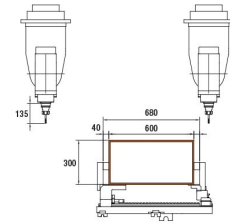
Centrum pro obrábění tyčí SBZ 151 Edition 90
