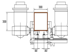
Centrum pro obrábění tyčí SBZ 151 Edition 90
